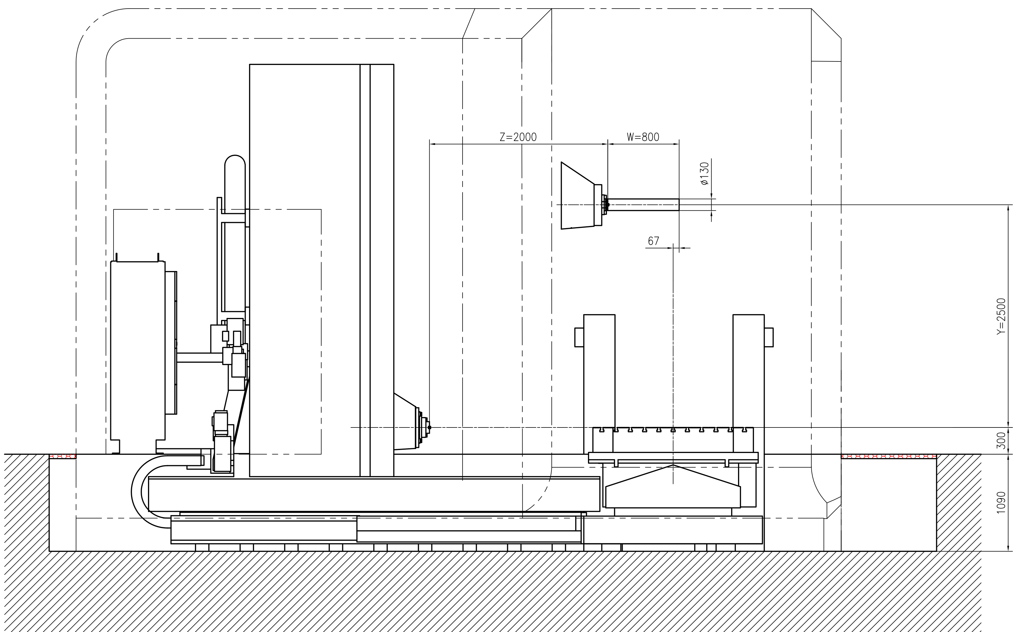
视图 A
